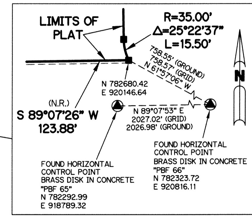
DETAIL "B" N.T.S.
